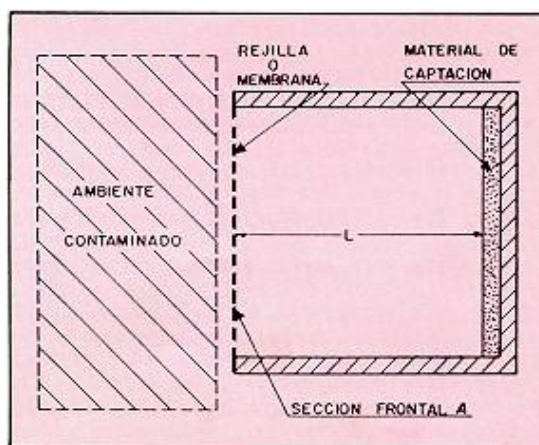
Fig. 1: Captador pasivo
