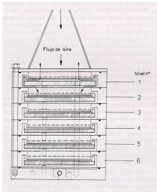
Fig. nº 2: Impactador inercial multinivel. Impactador Andersen
