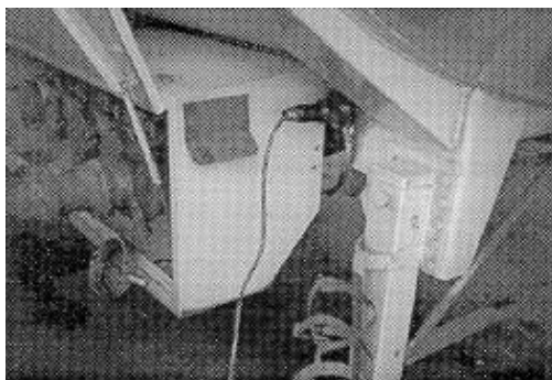
Fig. 4: Caja metálica de protección en la que se localizan las válvulas de carga. Contigua a esta caja se observa el dispositivo de conexión de la puesta a tierra
