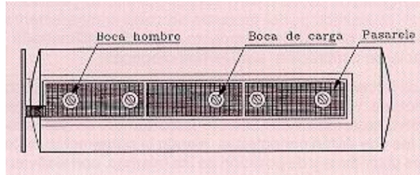
Fig. 6: Dispositivos en cúpula de cisterna correspondientes a bocas de hombro, bocas de carga y pasarela con plataforma de desembarco desde la escala de acceso
