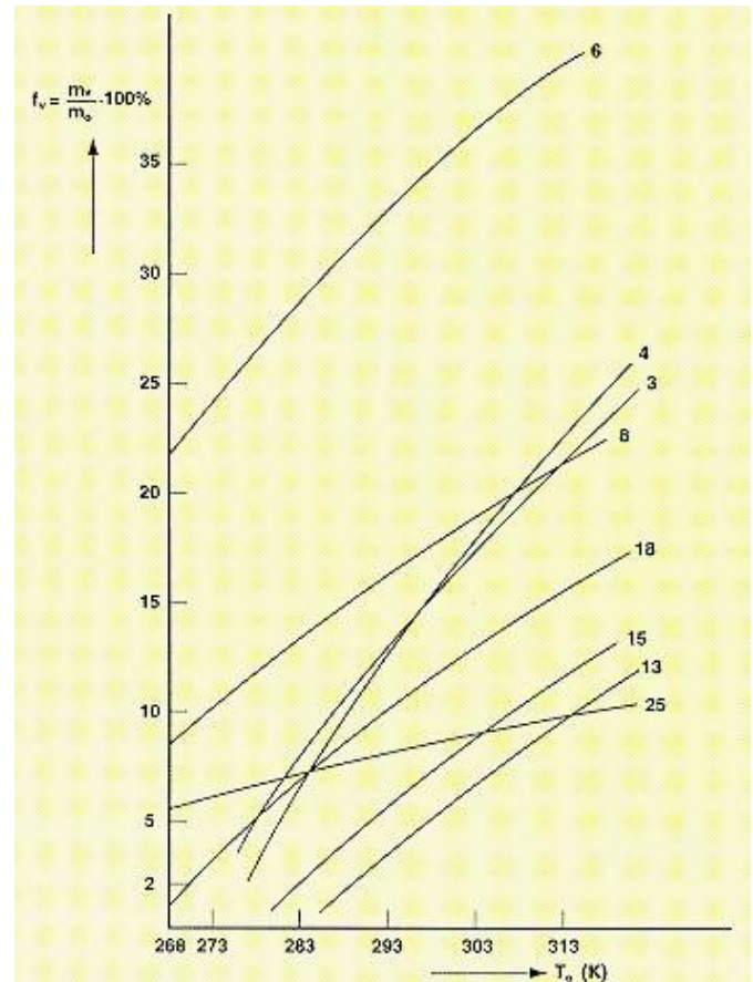
Fig. 2: Fracción teórica (calculada) vaporizada inicialmente en la expansión adiabática de un gas licuado a presión (número de referencia en tabla 1)
